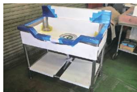
ステンレス製品の製作（シンク）
